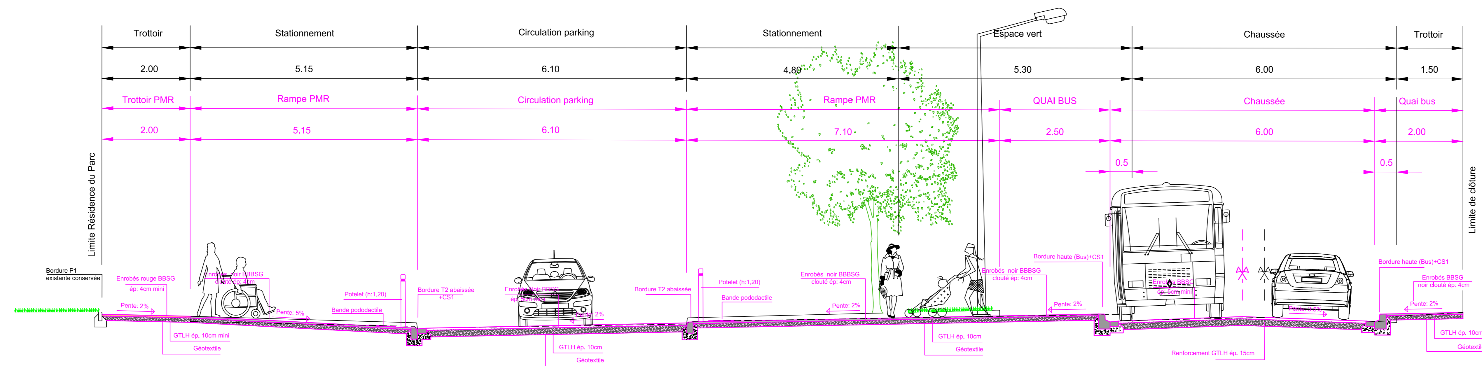
COUPE EN TRAVERS TYPE
